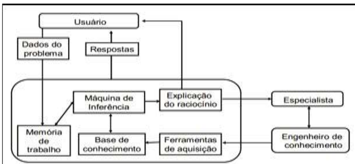
Quadro 2 - Sistemas Especialistas: Arquitetura
